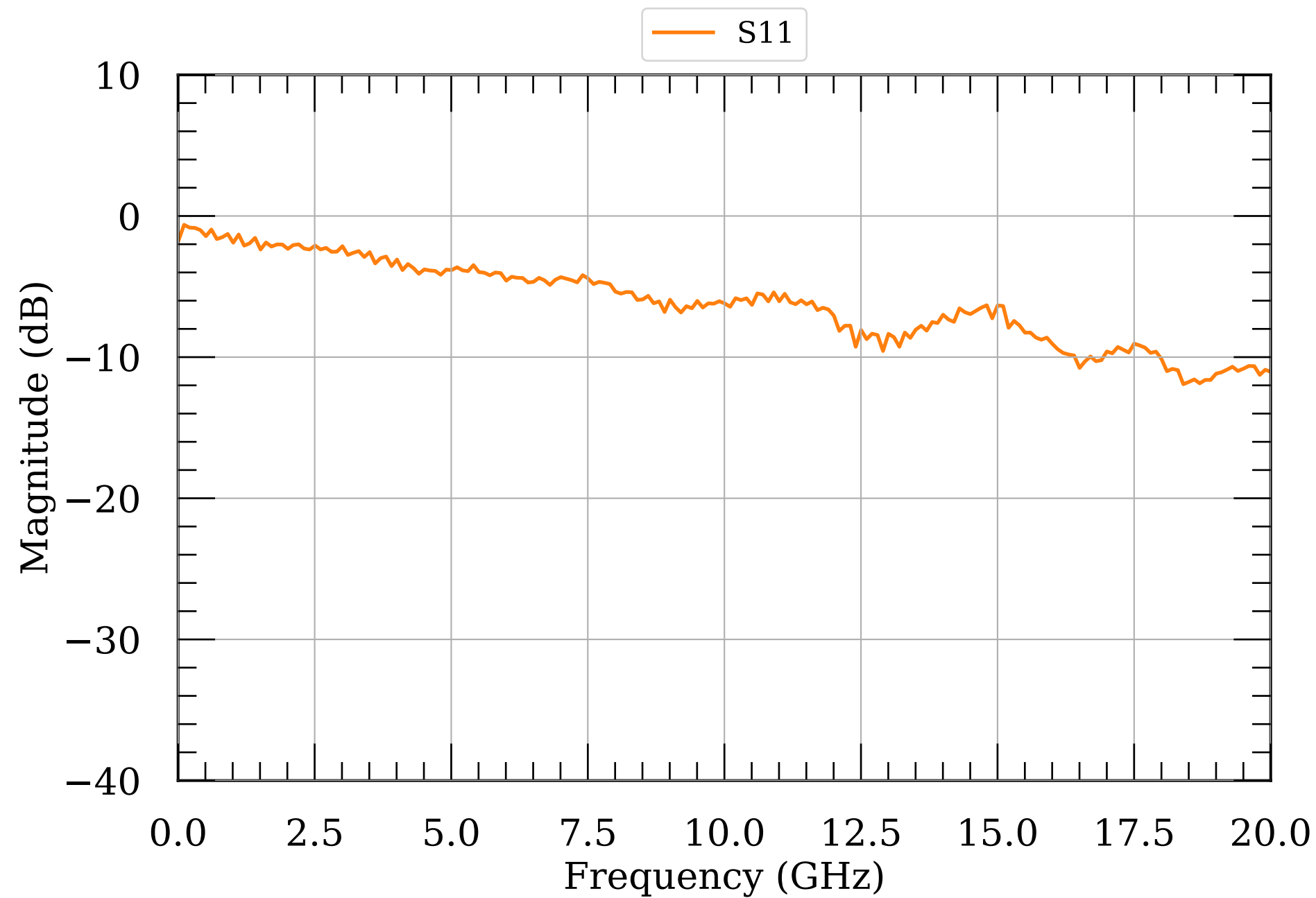
LNA S-params module028
